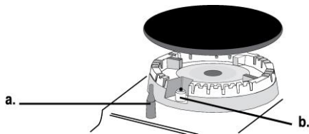
a. SICHERHEITSVORRICHTUNGEN b. Zündkerze der GASBRENNER
